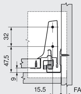
Cote de asamblare front pentru montare cu șuruburi
