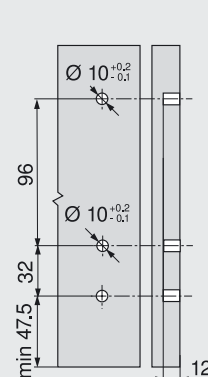
Cote de găurire front pentru EXPANDO
