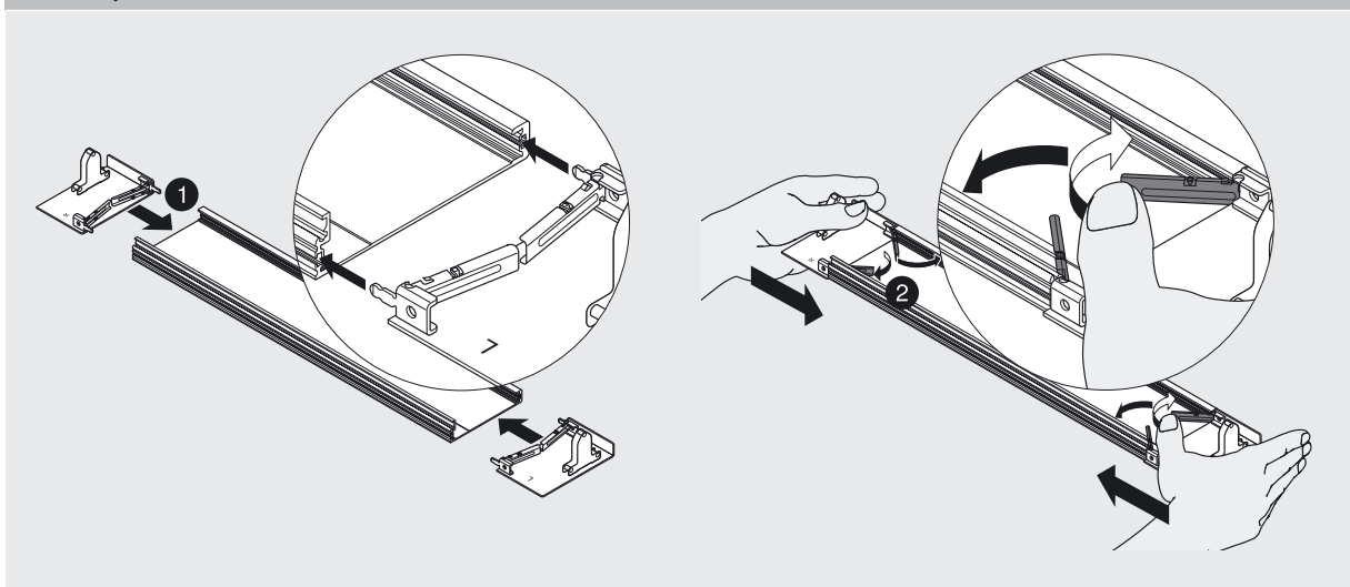
Montare piesă frontală
