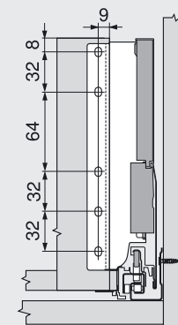
Cote de asamblare spate sertar
