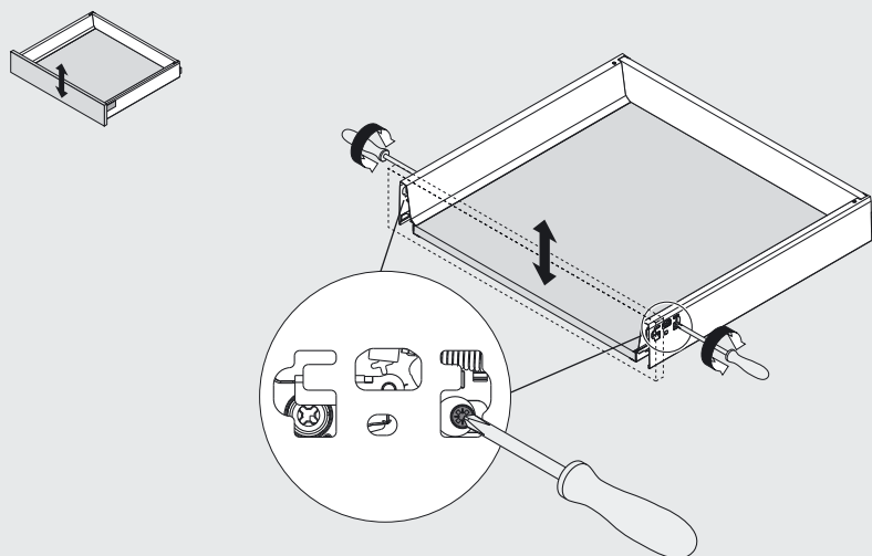
Reglare pe înălțime
