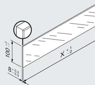
Cote de debitare element de inserție
