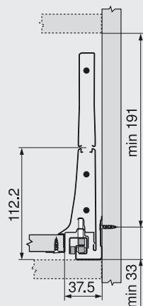
Cote de debitare pentru PAL de 16-mm
