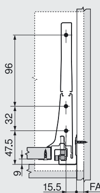
Cote de asamblare front pentru montare cu șuruburi
