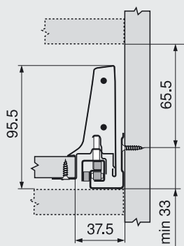
Spațiu necesar în corp
